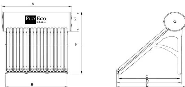
Rozmiary oraz wagi podgrzewaczy z serii PROECO HP
