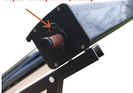
Miejsce na czujnik temperatury
