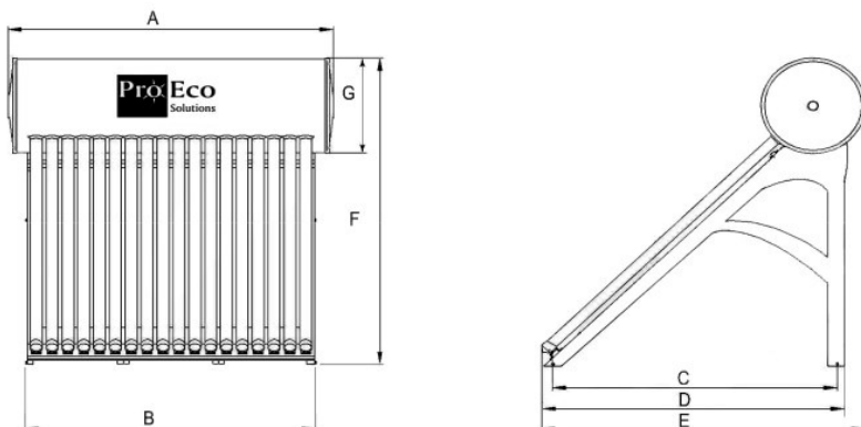
Rozmiary oraz wagi podgrzewaczy z serii PROECO YL
