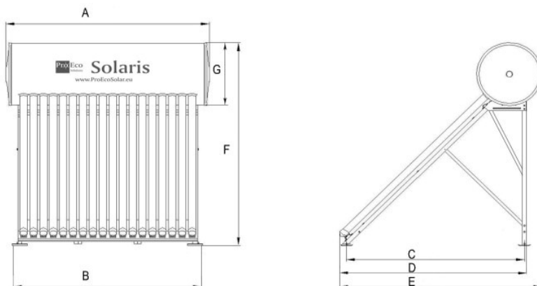
Rozmiary oraz wagi podgrzewaczy z serii PROECO SOLARIS – X
